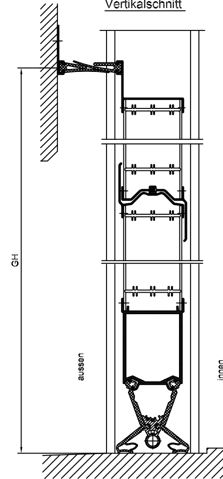
Vertikalschnitt
