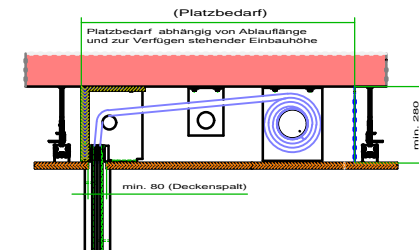
Sonderlösung für Einbau in Zwischendecke (Platzbedarf)
