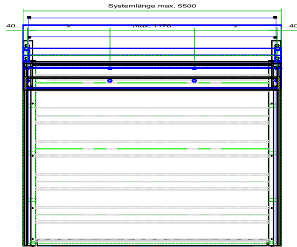
Horizontalschnitt
