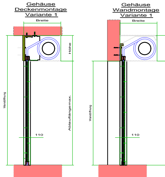
Vertikalschnitt
