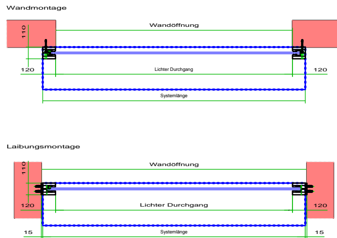
Horizontalschnitt
