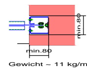
Seitliche Führung Nischenmontage
