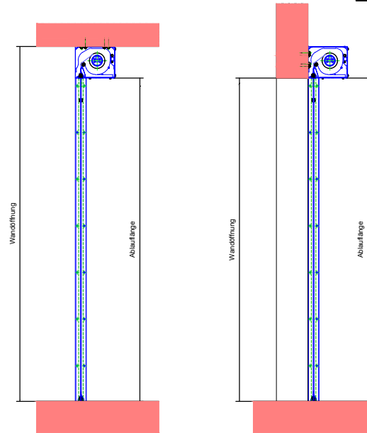
Seitliche Führung Wandmontage
