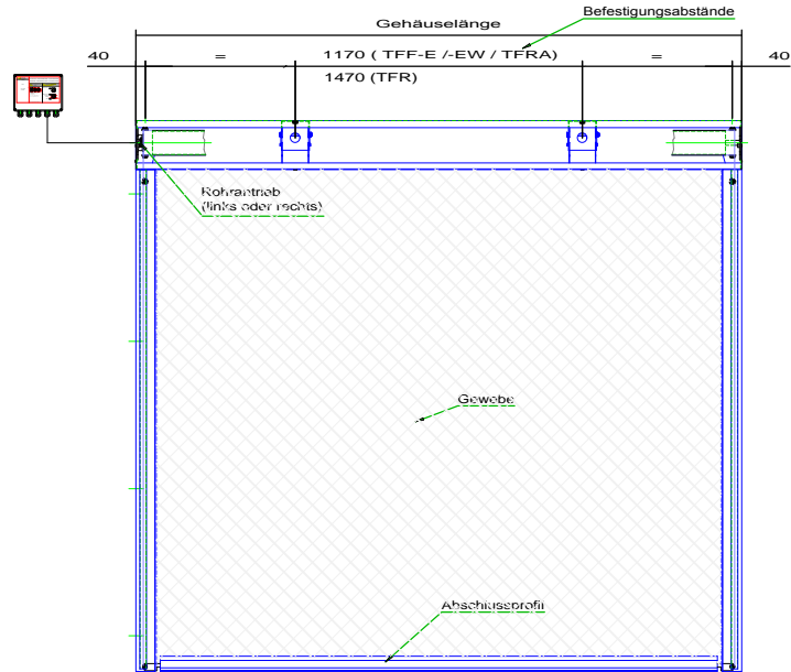
Ansicht
