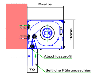
Gehäuse Wandmontage
