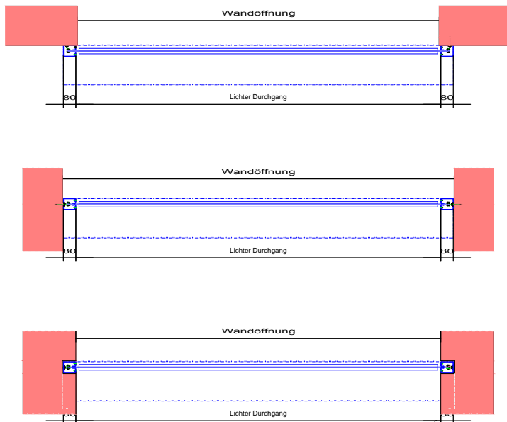
Horizontalschnitt
