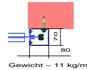
Seitliche Führung Laibungsmontage
