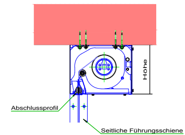
Gehäuse Deckenmontage
