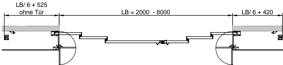
Horizontalschnitt
