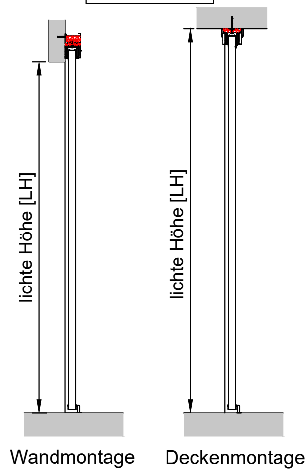
Vertikalschnitt
