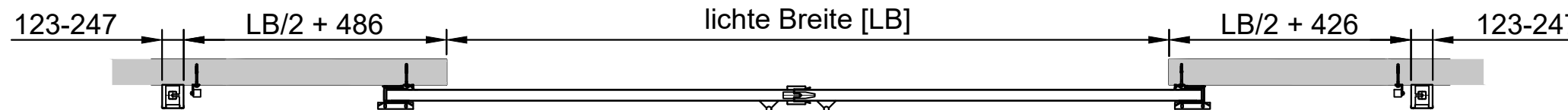
Horizontalschnitt
