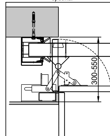
Seitenklappe "optional"
