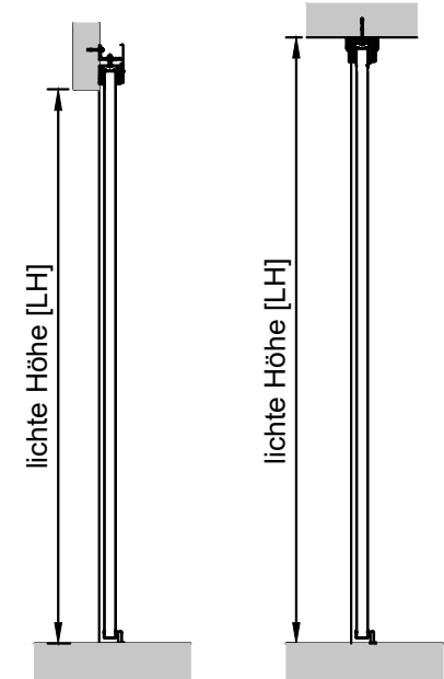
Vertikalschnitt
