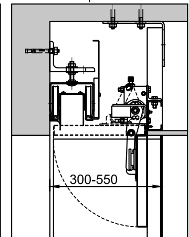
Deckenklappe "optional"
