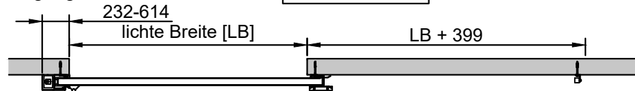
Gegengewicht umgelenkt
