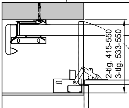
Seitenklappe "optional"
