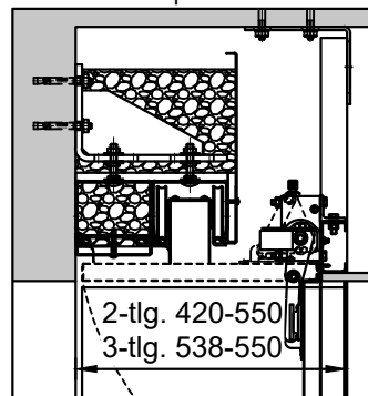
Deckenklappe "optional"
