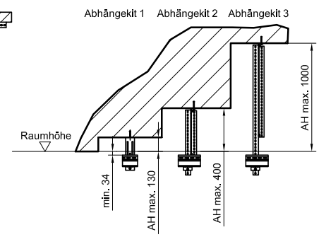
Detail Abhängekits
