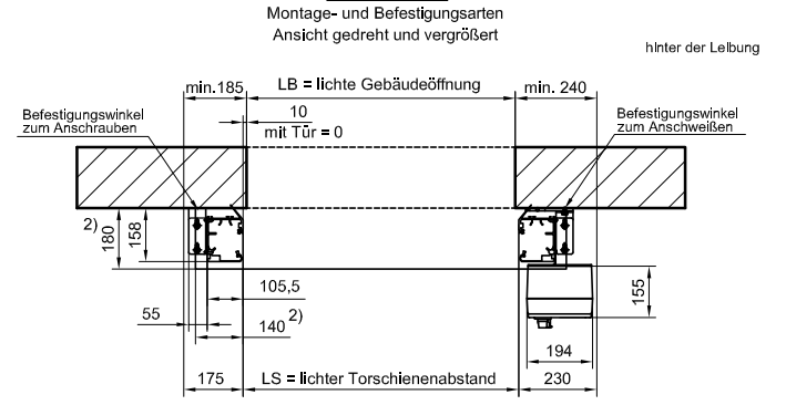
Schnitt D-D
