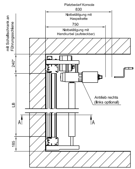
Schnitt B-B Tor geschlossen
