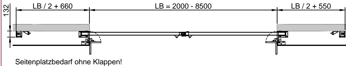
Horizontalschnitt
