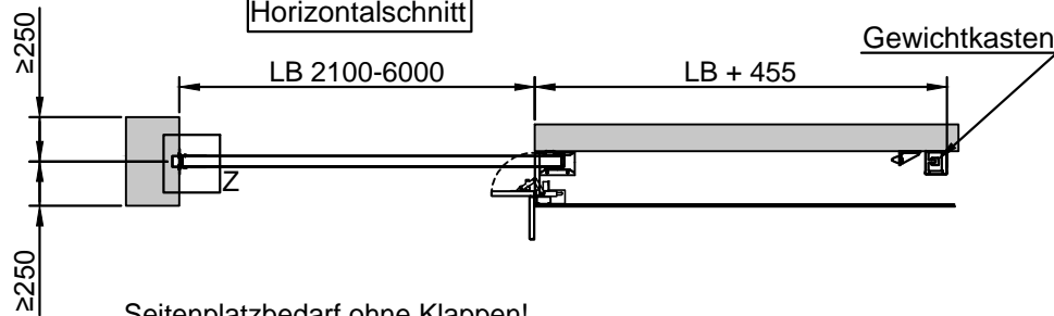
Horizontalschnitt
