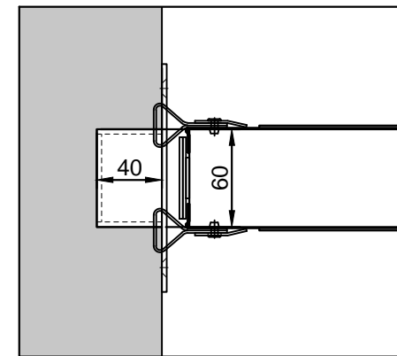
Detail Z Wandhülse 60x80x40
