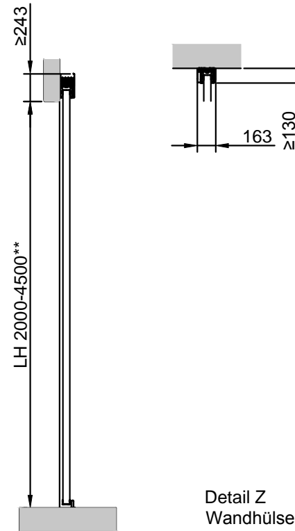
Vertikalschnitt
