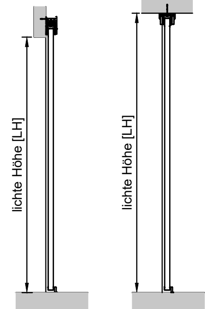
Vertikalschnitt
