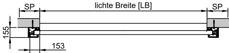
Horizontalschnitt
