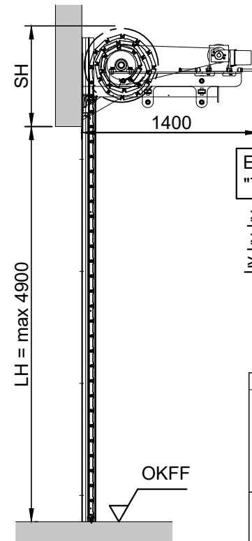
Vertikalschnitt
